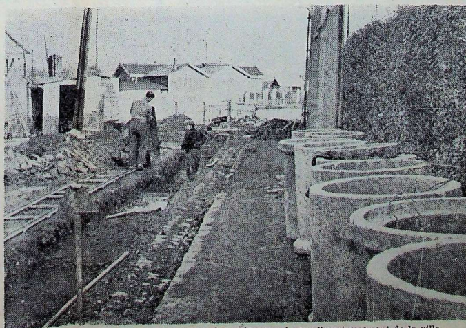
La Municipalité a décidé d'établir un plan quinquennal pour l'assainissement de la ville. Les premiers travaux pour l'année 1954 viennent de commencer rue Galliéni et sont menés à un rythme accéléré sous la direction de l'ingénieur des Ponts-et-Chaussées VANDENBERGUE. Sur notre photo, les ouvriers percent les tranchées pour la pose des nouveaux aqueducs. Dans quelques mois la rue sera recouverte de tarmac.
